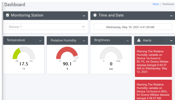
Fig. 16. Dashboard module.
