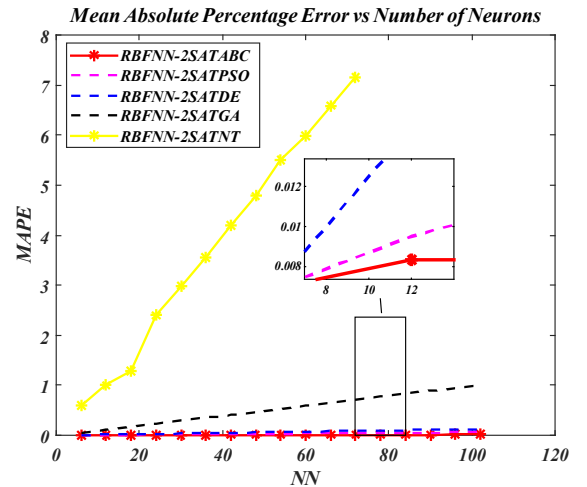
Fig. 7. MAPE evaluation.
