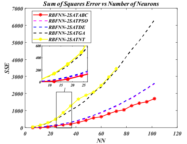
Fig. 6. SSE evaluation.
